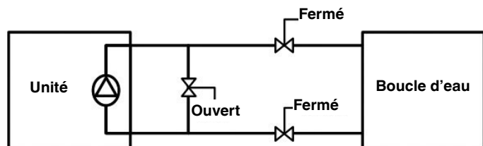
Figure 26 : Position hiver pour unité avec module hydraulique
