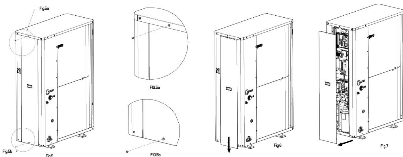
Figure 5 : Retrait du panneau latéral droit
