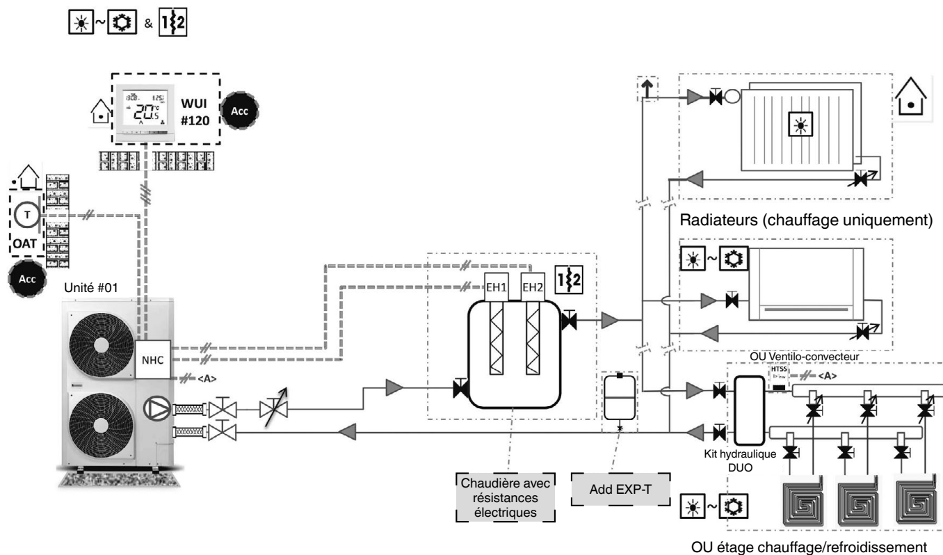
Figure 13 : Installation standard avec résistances électriques de chauffage additionnel
