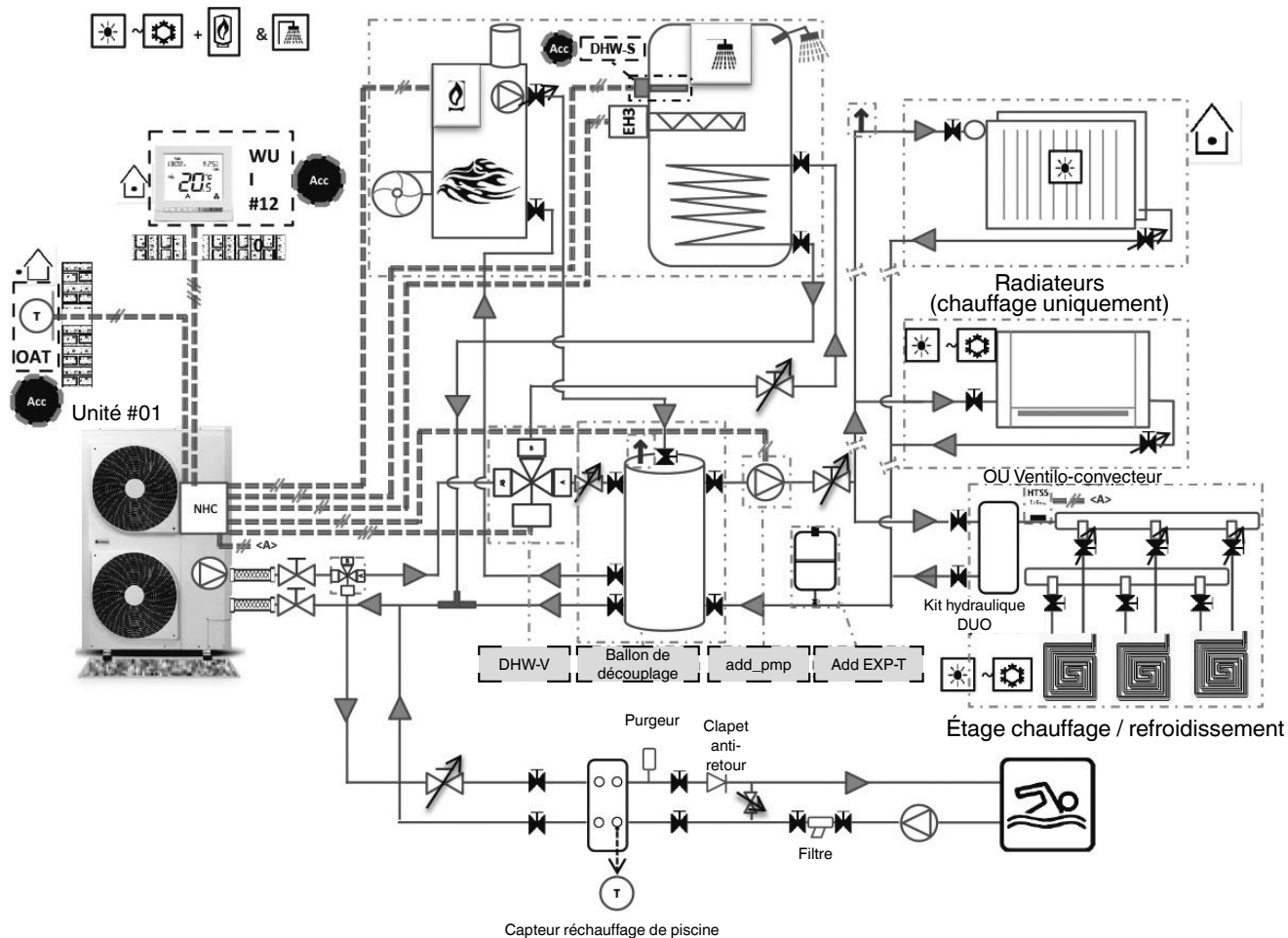
Figure 19 : Installation standard avec production d'ECS, chauffage piscine et chauffage d'ambiance (chauffage au sol ou radiateur/ventilo-convecteur)
