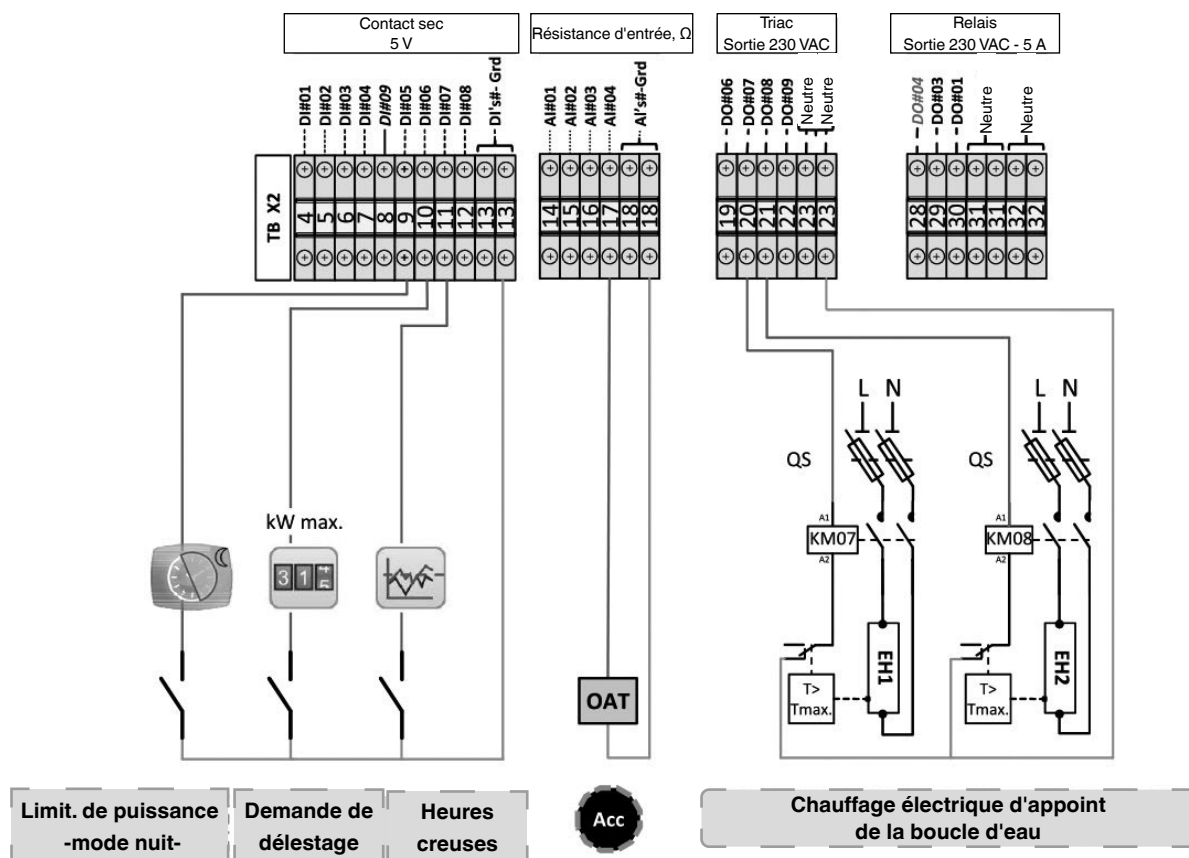
Figure 14 : Branchement électrique sur le bornier pour les résistances électriques de chauffage additionnel
