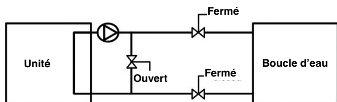
Figure 27 : Position hiver pour unité sans module hydraulique
