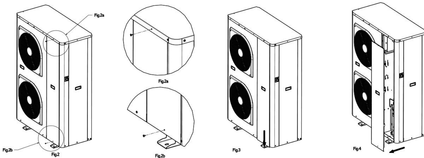
Figure 5 : Retrait du panneau latéral droit
