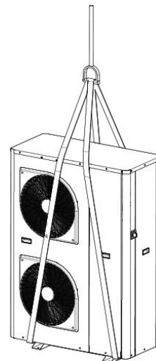
Figure 3 : Configuration pour l'installation
