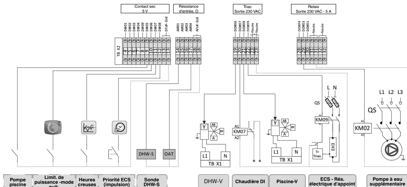
Figure 20 : Branchement électrique sur le bornier pour la production d'ECS, le chauffage ambiant, la production de chauffage pour piscine et la chaudière
